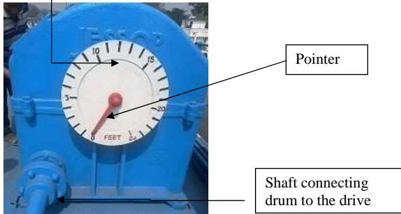
Fig. 3 Display Dial
